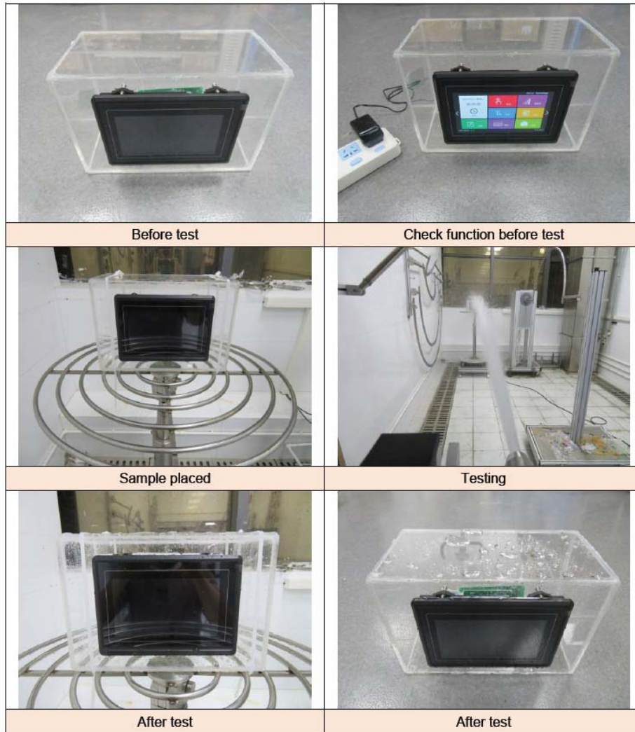
图 6-8 防水测试图
